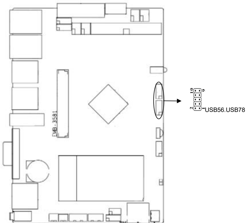
J12: OTG 烧录程序, DEBUG 调试串口 2*5PIN 2.00mm 排针
