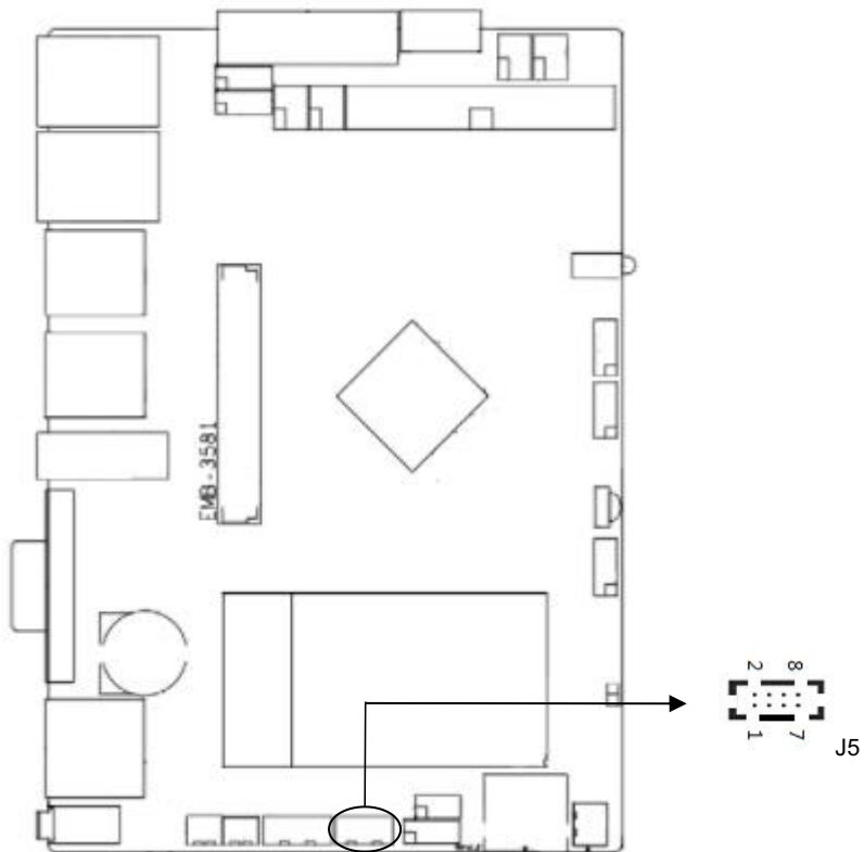
J5: 2*4PIN 2.00MM 小白座
