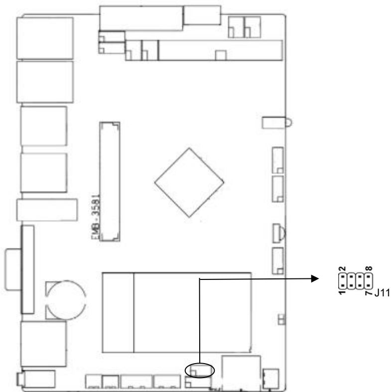
J11: 按键（烧录跳冒）
