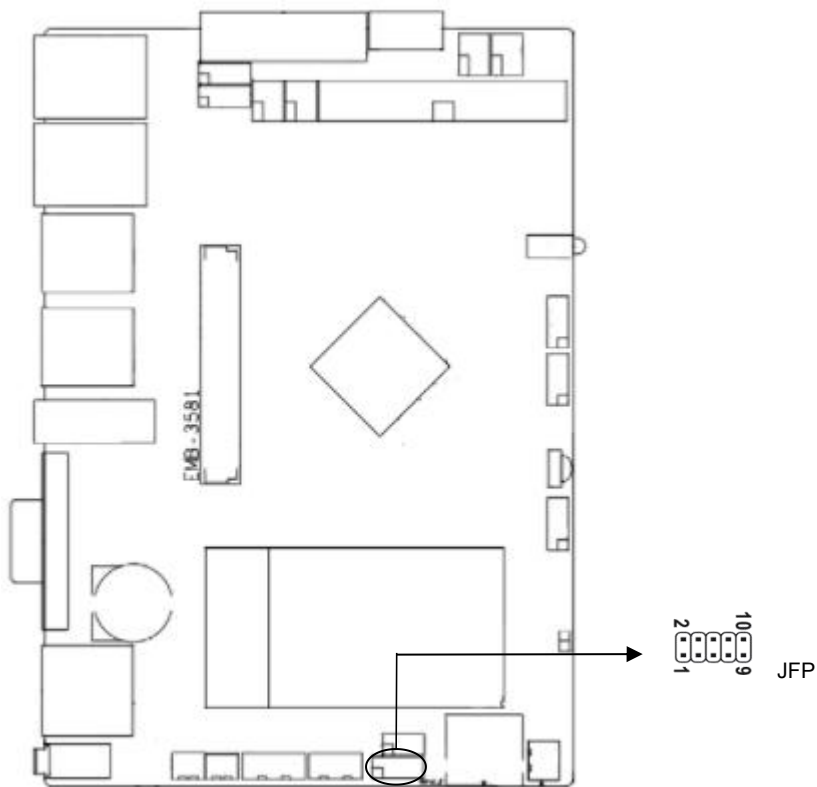
JFP: 2*5PIN 2.00MM排针
