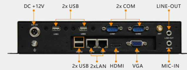
后面板接口
