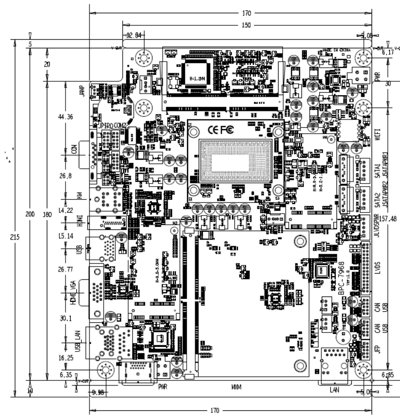
BPC-7968 接口位置和尺寸图
