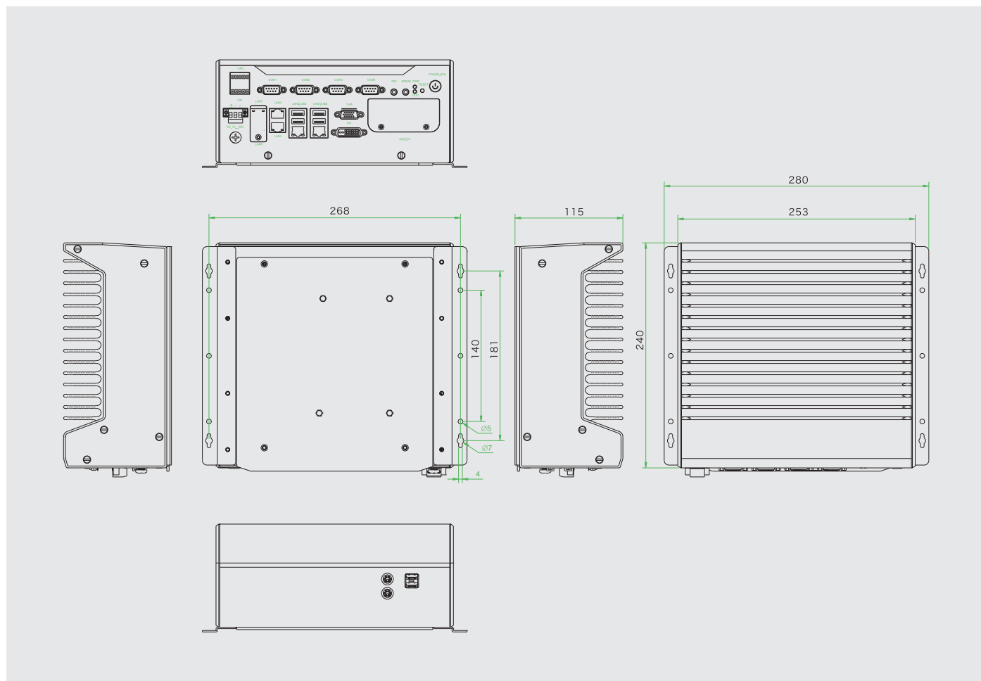
尺寸图:
